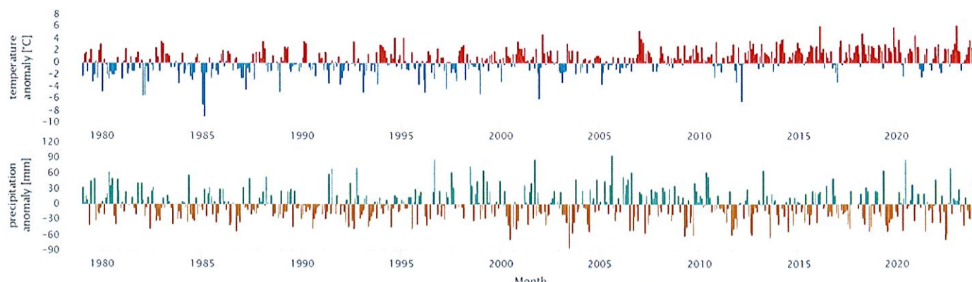
Figura 37. Dinamica anomaliilor lunare de temperatură și precipitații din zona de studiu 51
