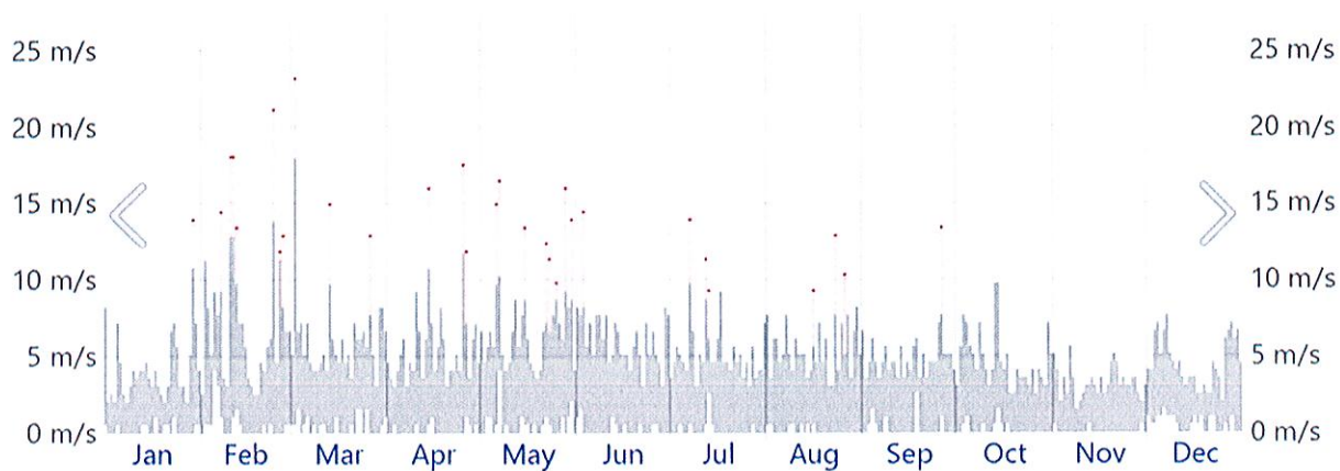
Figura 38d. Viteza vântului în anul 2020
