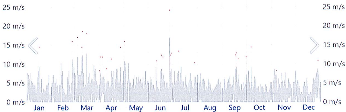
Figura 38e. Viteza vântului în anul 2019
